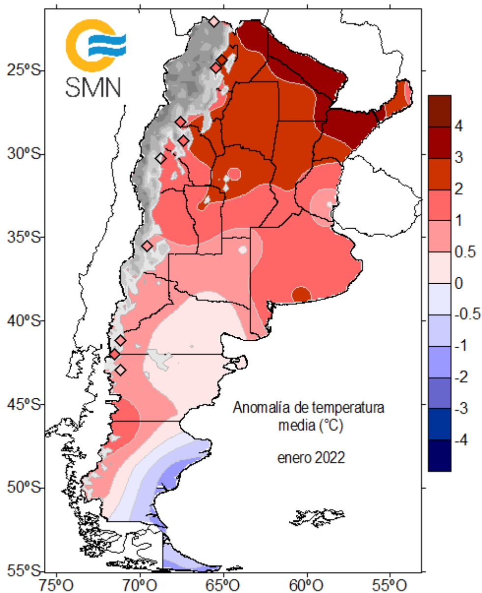
Figura 1 Mapa con las anomalías respecto a la climatología de todo enero 2022.
