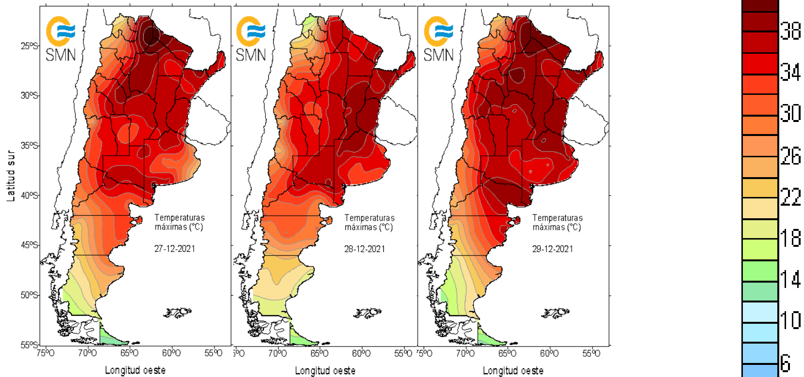
Figura 2 Mapas de temperaturas máximas del 27 al 29 de diciembre 2021, valores en grados Celsius (escala a la derecha). Fuente: SMN.
