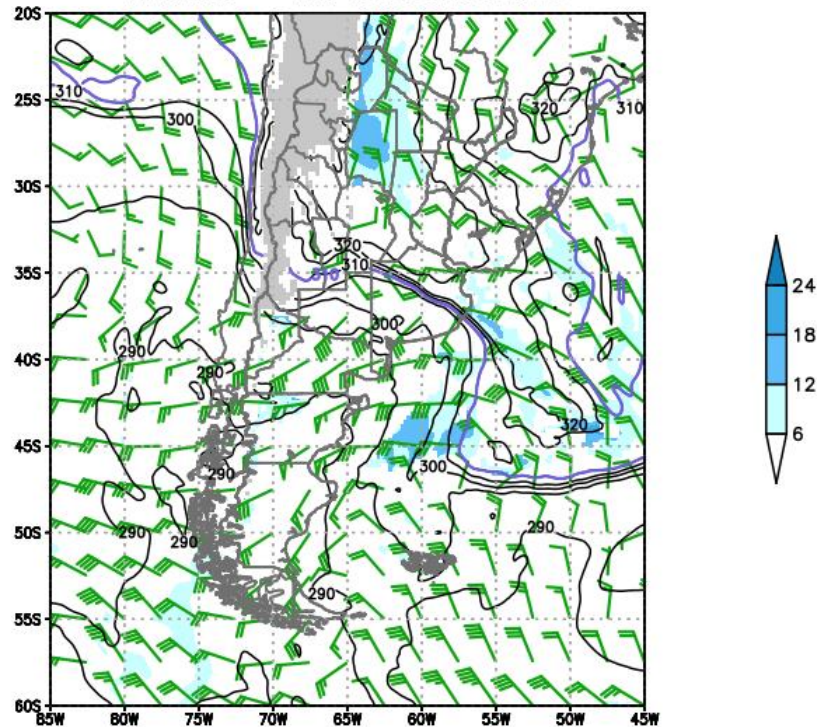
Figura 6. Viento en el nivel de 850 hPa, Criterio de Bonner (tonos azulados) y temperatura potencial equivalente para igual nivel de presión, temperatura geopotencial equivalente en el nivel de 850 hPa con viento en dicho nivel para el 06 de agosto de 2020 respectivamente de las 00 Z. Para mayores detalles de unidades y otros ver escritos en los mapa. Fuente: basado en análisis del modelo GFS, procesado por Dcao / Cima.
