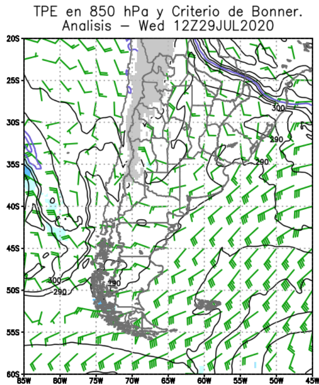
Figura 5. Viento en el nivel de 850 hPa, Criterio de Bonner (tonos azulados) y temperatura potencial equivalente para igual nivel de presión, temperatura geopotencial equivalente en el nivel de 850 hPa con viento en dicho nivel para el 29 de julio de 2020 respectivamente de las 12 Z. Para mayores detalles de unidades y otros ver escritos en los mapa.
