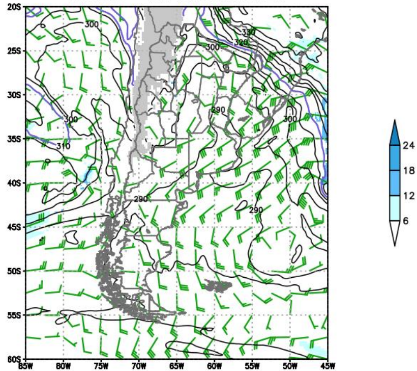
Figura 3. Viento en el nivel de 850 hPa, Criterio de Bonner (tonos azulados) y temperatura potencial equivalente para igual nivel de presión, para el 26 de junio 2020 a las 0 Z.
