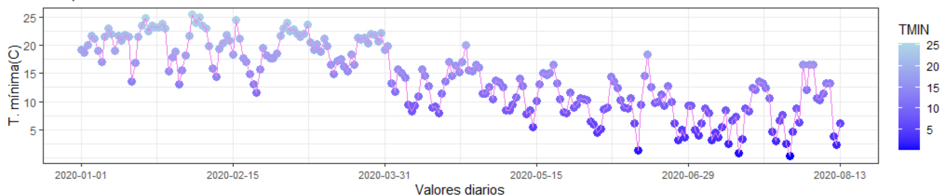
Figura 1 Temperaturas máximas y mínimas diarias durante enero al 13 de agosto de 2020 para el Observatorio Central Buenos Aires. Formato eje de abscisas con la fecha: año, mes y día. Elaborado con datos preliminares del SMN.
