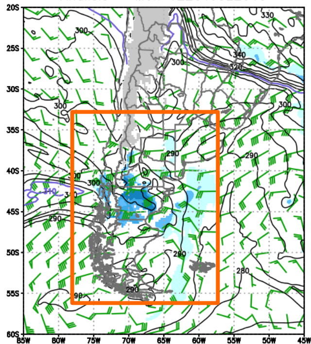
TPE en 850 hPa y Criterio de Bonner. Analisis – Mon 12Z01JUL2019
