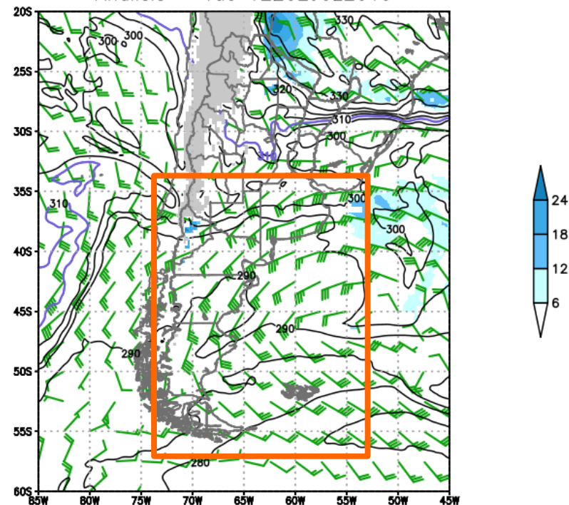
TPE en 850 hPa y Criterio de Bonner. Analisis – Tue 12Z02JUL2019
